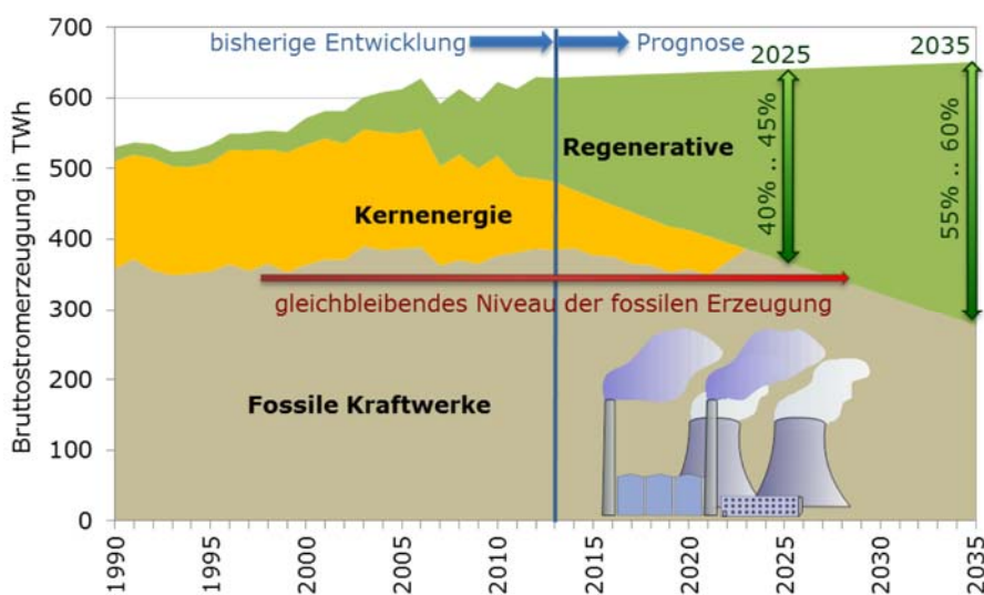
Abbildung 4: Prognose der Entwicklung der Stromerzeugung in Deutschland bei Umsetzung des Zielkorridors für erneuerbare Energien der Bundesregierung [Qua14]
