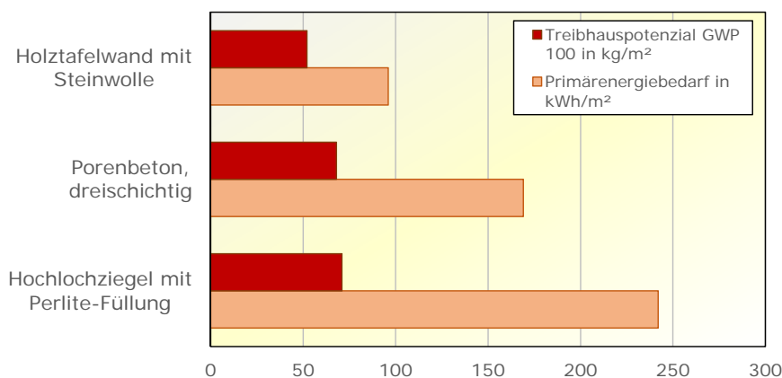
Abbildung 6: Ökobilanz verschiedener Außenwandtypen (Daten: [Oeh12])
