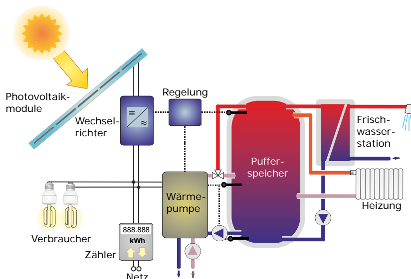
Abbildung 8: Photovoltaisch unterstütztes Wärmepumpensystem
