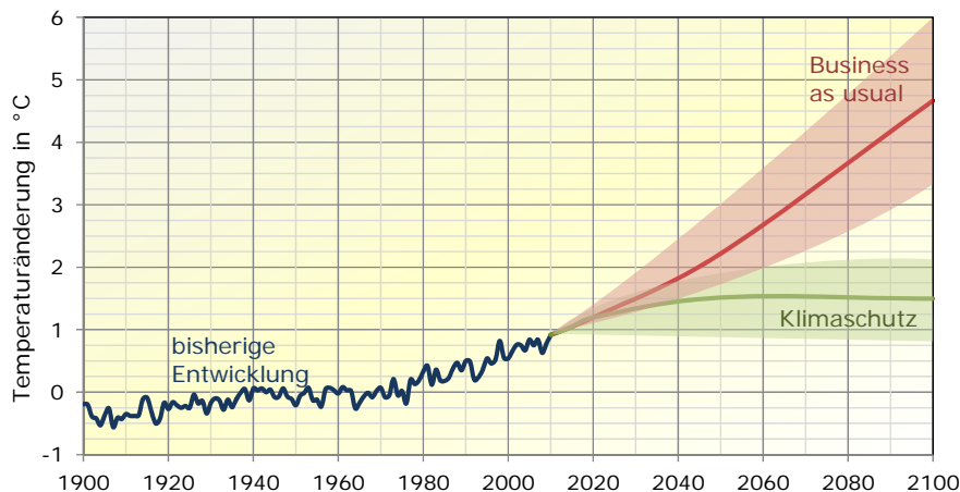
Abbildung 2: Entwicklung der mittleren globalen Oberflächentemperatur im Vergleich zum Mittelwert der Jahre 1951 bis 1980 für zwei verschiedene Szenarien. (Daten: [NAS13, IPC13])
