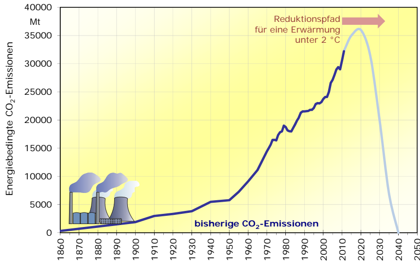
Abbildung 1: Reduktionspfad für die weltweiten Kohlendioxidemissionen zur Begrenzung der globalen Erwärmung auf weniger als 2°C (Daten [WBG08]).
