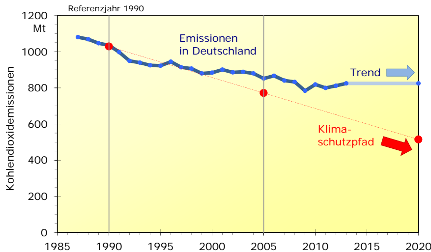
Abbildung 3: Entwicklung der energiebedingten Kohlendioxidemissionen in Deutschland im Vergleich zu den Erfordernissen für einen wirksamen Klimaschutz
